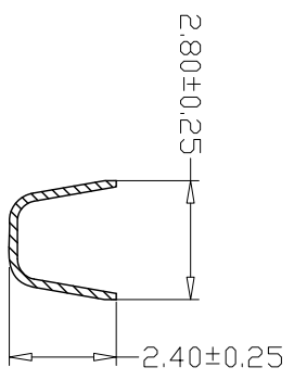
SEC: A-A
